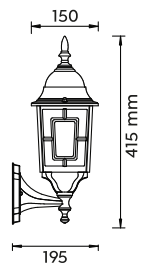
Sockelleuchte · Podestal lamp excl. 1 x E27 max. 60 W 505960128
