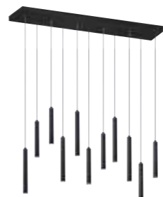
Pendelleuchte · Pendant ↔ 115 x 15 cm, ↑ 150 cm incl. 11 x SMD-LED, 2,8 W 11 x 350 lm, 3.000 K
